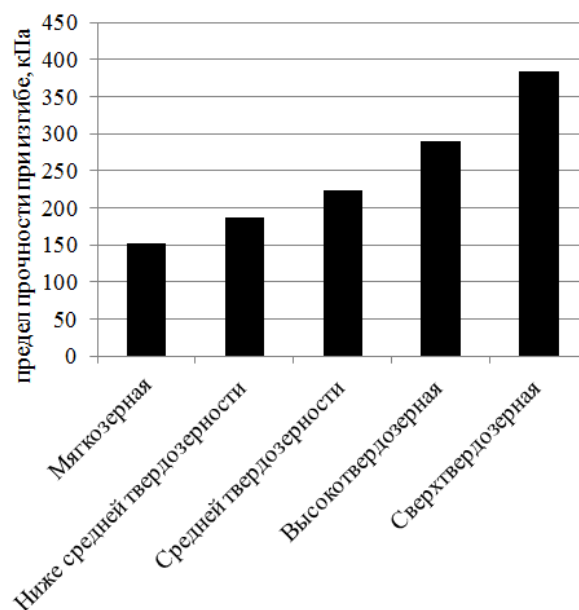
Рис. 1. Варьирование предельной прочности на изгиб образцов сахарного печенья в зависимости от степени твердозерности пшеницы
