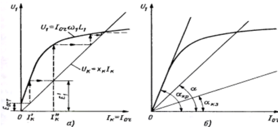
Рис. 3. Самовозбуждение асинхронного генератора с остаточным полем ротора: а – графическое изображение процесса самовозбуждения, б – характеристики намагничивания
