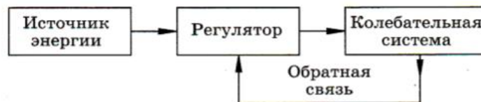
Рис. 6. Типовая структурная схема автоколебательной системы
