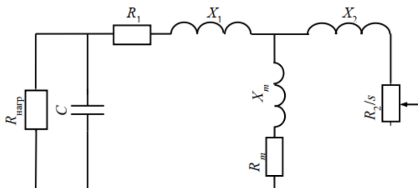
Рис. 4. Схема замещения асинхронного генератора с конденсаторной батареей
