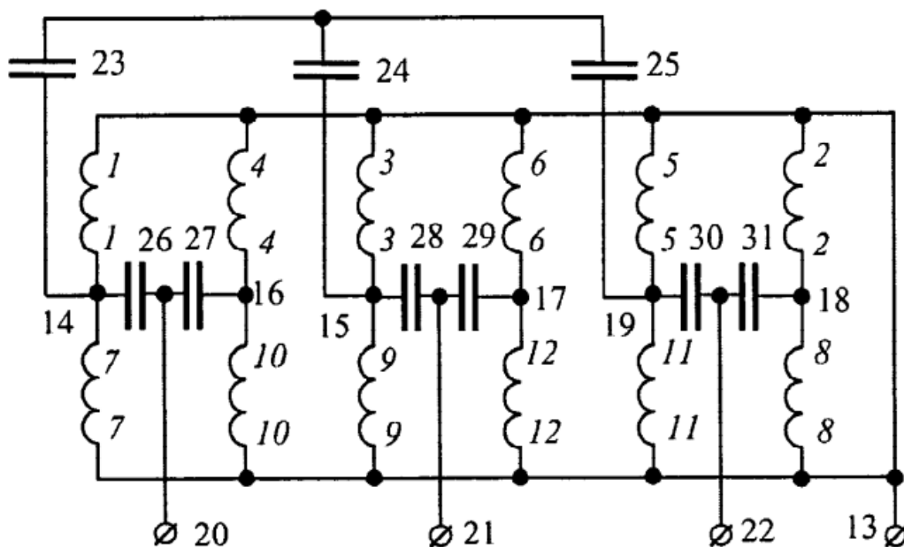
Рис. 2. Схема обмоток
